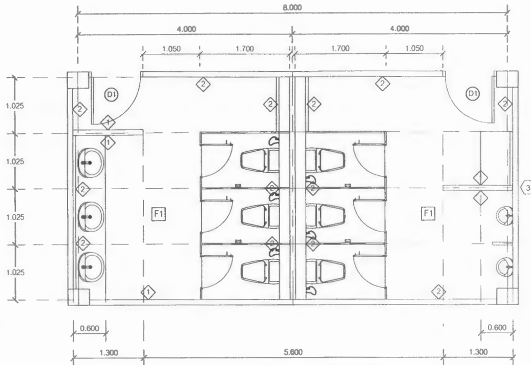
รายละเอียดเนื้องานปรับปรุงห้องน้ำชาย-หญิง ชั้น 1 - ชั้น 4 เดิม
