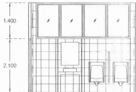
รูปตัด D - D scale 1:50
