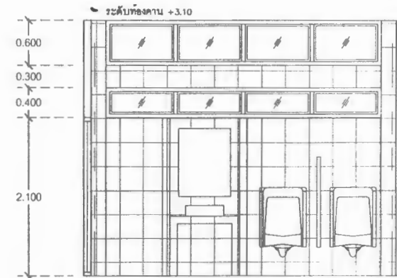
รูปตัด C - C scale 1:50
