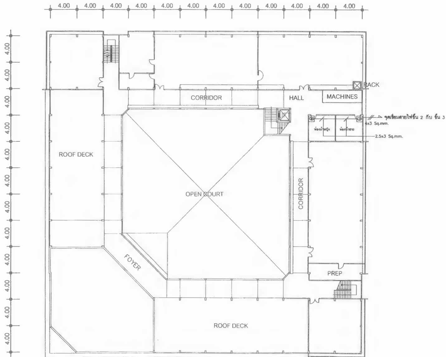
ผังเมนไฟฟ้าชั้น 3 อาคารบริหารหลังเก่า SCALE 1:250
