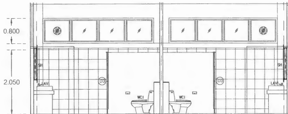
รูปตัด A - A scale 1:50
