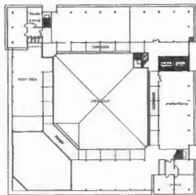
ผังบริเวณปรับปรุงห้องน้ำชั้น 4
