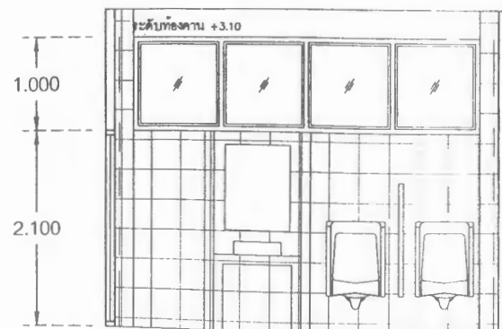
รูปตัด E - E scale 1:50
