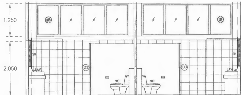
รูปตัด B - B scale 1:50
